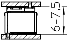
FP 0,8/..-FV-SH 4,85
