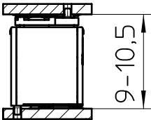
FP 0,8/..-FV-SH 7,85
