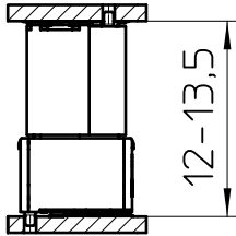
FP 0,8/..-FV-SH 4,85
