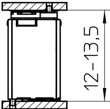
FP 0,8/..-FV-SH 10,85
