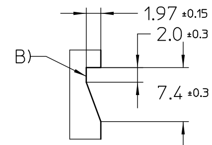
Detail1 2:1
