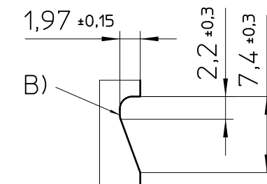
Detail1 2:1
