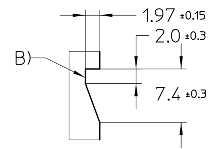
Detail1 2:1
