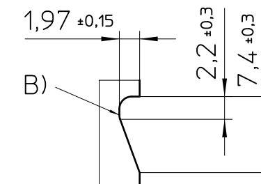
Detail1 2:1
