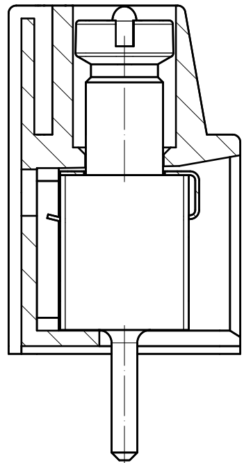
A-A
