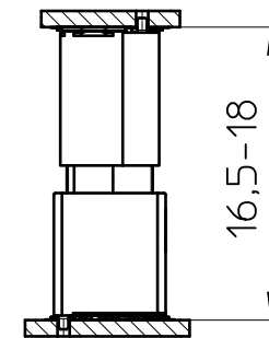
FP 0,8/..-FV 7,85
