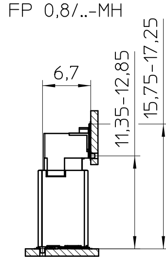
FP 0,8/..-FV 10,85
