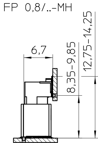
FP 0,8/..-FV 7,85
