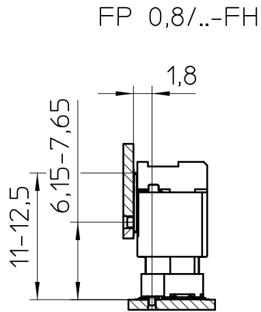
FP 0,8/..-MV 2,65
