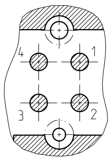
X Pinbelegung 3:1 (Buchse)
