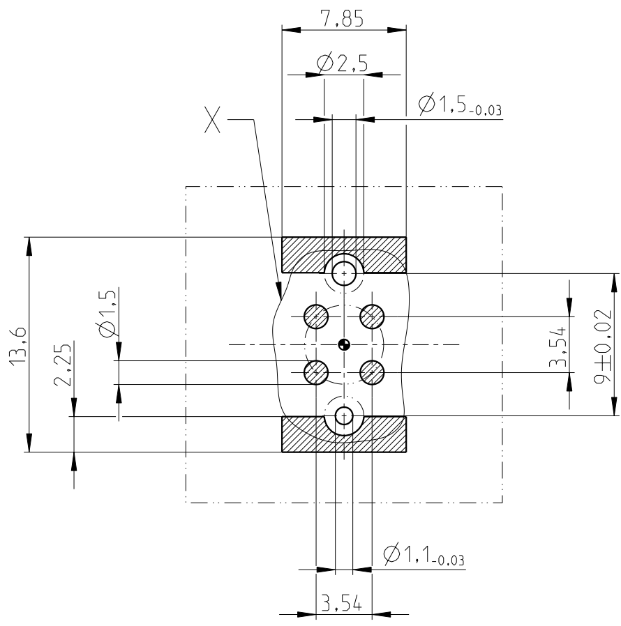
X Pinbelegung 3:1 (Stift)
