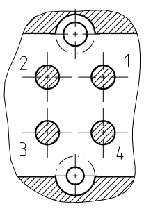
X Pinbelegung 3:1 (Stift)
