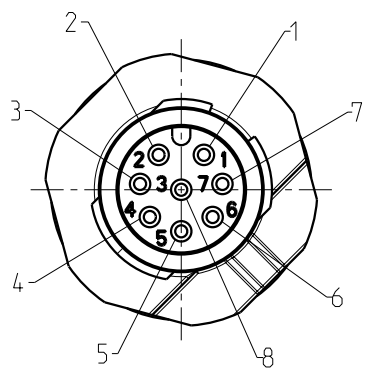
Ansicht Polbild Steckseite
