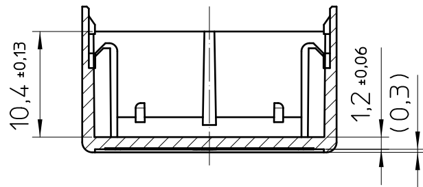
A-A 2:1
