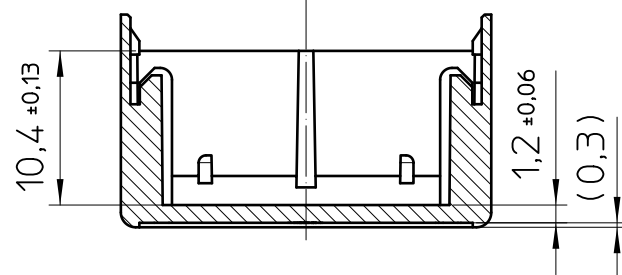
A-A 2:1
