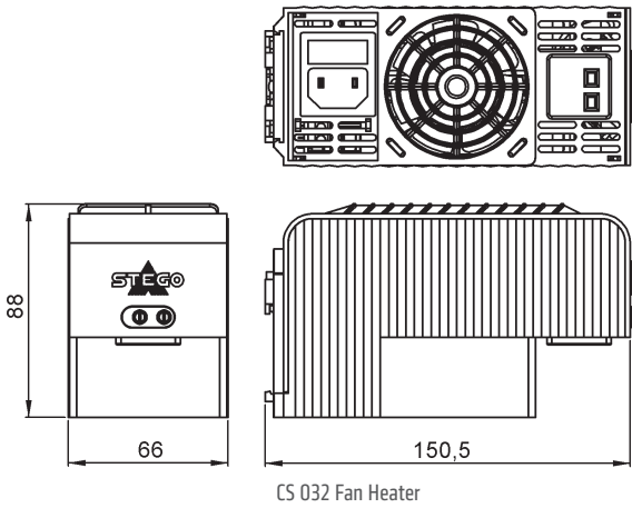
CS 032 Fan Heater
