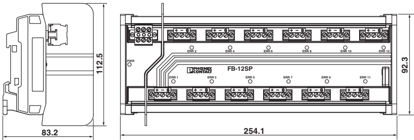
Figure 2 FB-8SP, FB-12SP
