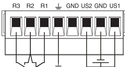
Bild 4 Anschluss einer einzigen Spannungsversorgung
