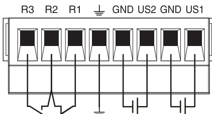
Bild 3 Anschluss einer redundanten Spannungsversorgung
