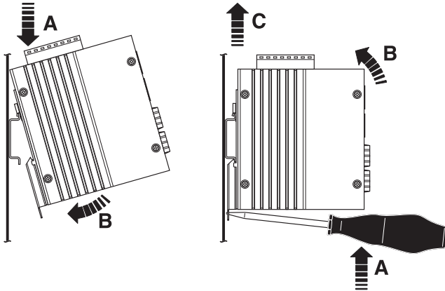
Bild 2 Montage/Demontage
