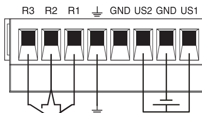
Figura 4 Connessione di un'alimentazione di tensione singola
