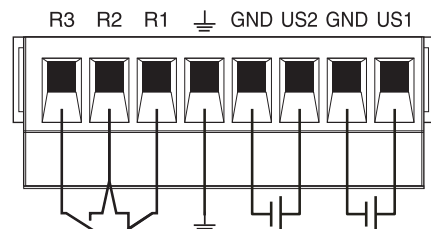
Figura 3 Connessione di un'alimentazione di tensione ridondante
