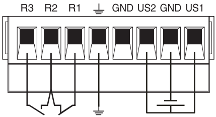
图 4 单独电源连接
