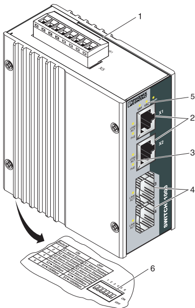
图 1 连接器和 LED
