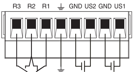
图 3 冗余电源连接
