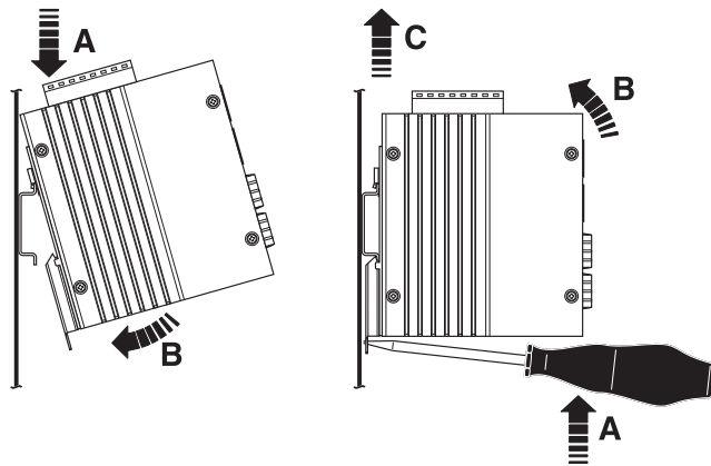
Bild 2 Montage/Demontage
