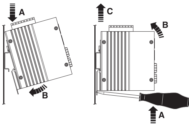
Рисунок 2 Монтаж/демонтаж
