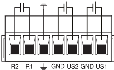
图 3 冗余电源连接
