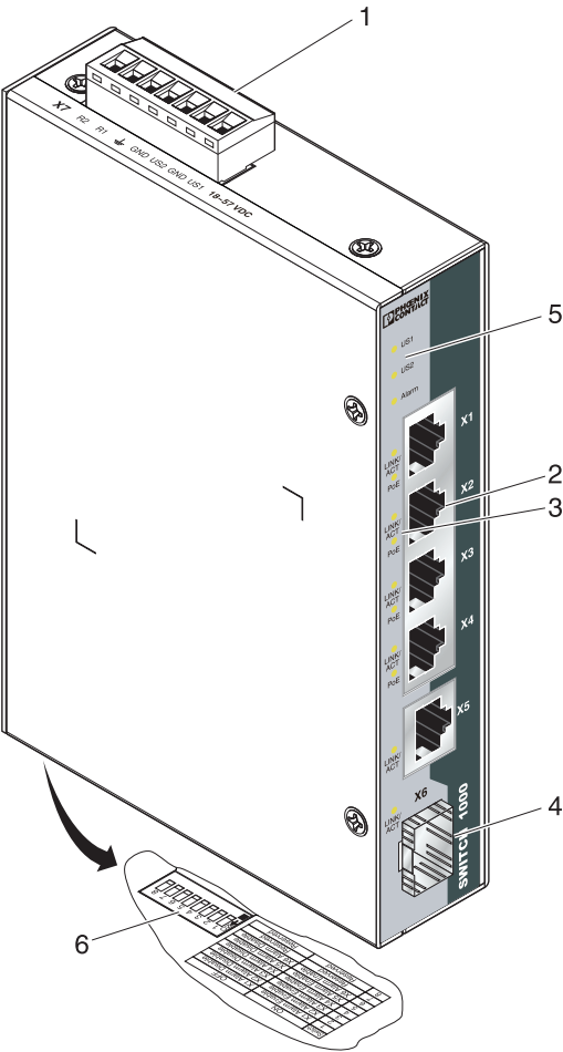
图 1 连接器和 LED
