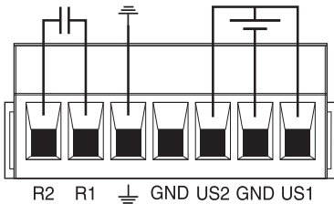
图 4 单独电源连接
