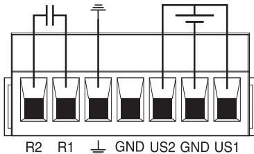
Рисунок 4 Подключение единственного источника питания
