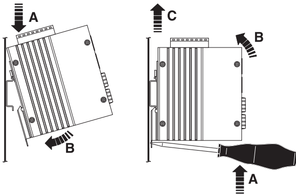
Рисунок 2 Монтаж/демонтаж
