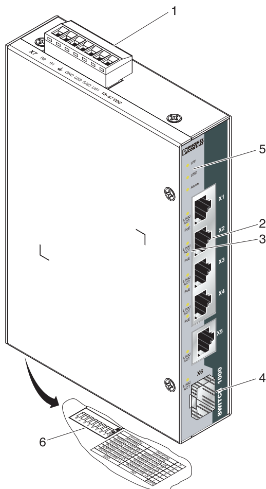
Рисунок 1 Соединители и светодиоды
