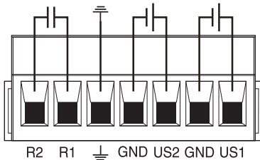
Рисунок 3 Подключение резервного источника питания
