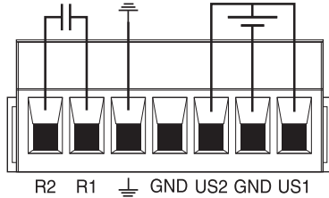
Şekil 4 Tek güç kaynağı bağlantısı
