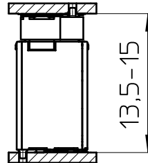
FP 0,8/..-FV-SH 10,85
