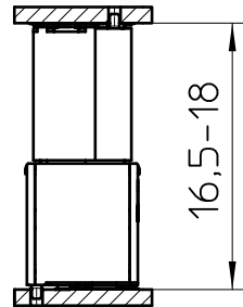
FP 0,8/..-FV-SH 7,85
