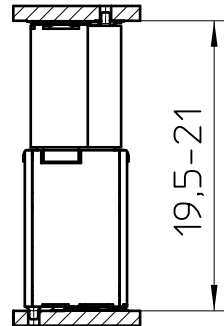
FP 0,8/..-FV-SH 10,85
