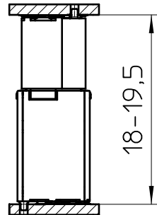
FP 0,8/..-FV-SH 10,85
