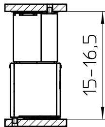
FP 0,8/..-FV-SH 7,85
