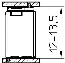
FP 0,8/..-FV-SH 10,85
