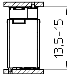
FP 0,8/..-FV-SH 10,85
