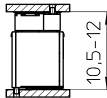
FP 0,8/..-FV-SH 7,85
