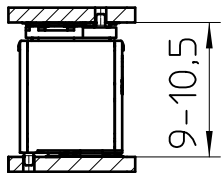
FP 0,8/..-FV-SH 7,85
