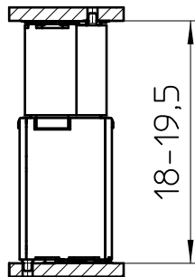
FP 0,8/..-FV-SH 10,85
