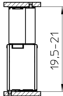
FP 0,8/..-FV-SH 10,85
