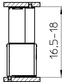
FP 0,8/..-FV-SH 7,85
