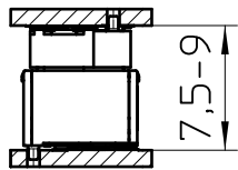
FP 0,8/..-FV-SH 4,85
