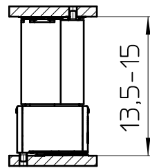
FP 0,8/..-FV-SH 4,85
