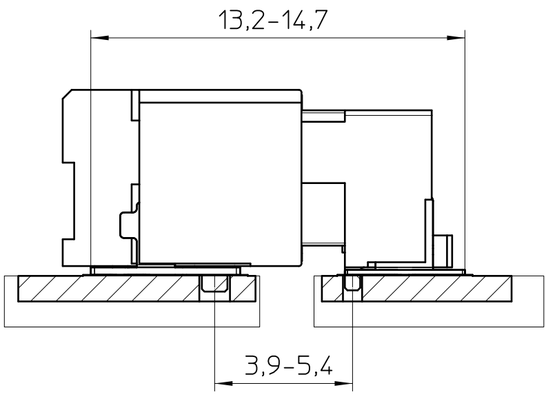
FP 0,8/..-FH FP 0,8/..-MH(-SL)
