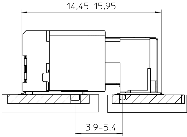
FP 0,8/..-FH-SH FP 0,8/..-MH-SH
