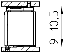
FP 0,8/..-FV-SH 7,85
