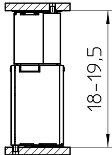
FP 0,8/..-FV-SH 10,85
