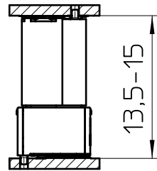
FP 0,8/..-FV-SH 4,85
