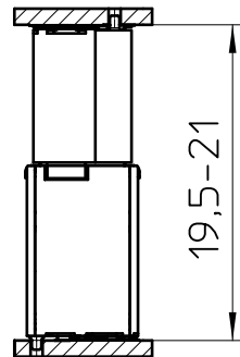
FP 0,8/..-FV-SH 10,85
