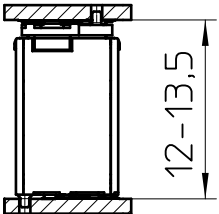
FP 0,8/..-FV-SH 10,85
