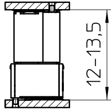
FP 0,8/..-FV-SH 4,85
