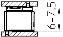
FP 0,8/..-FV-SH 4,85
