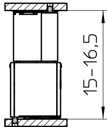
FP 0,8/..-FV-SH 7,85
