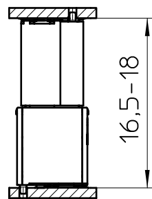
FP 0,8/..-FV-SH 7,85
