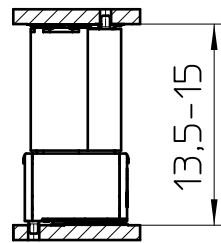
FP 0,8/..-FV-SH 4,85
