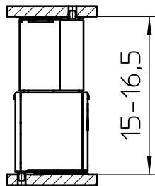
FP 0,8/..-FV-SH 7,85
