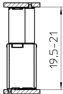
FP 0,8/..-FV-SH 10,85
