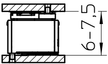
FP 0,8/..-FV-SH 4,85
