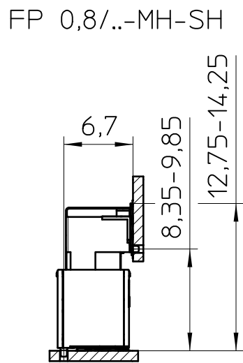
FP 0,8/..-FV-SH 7,85
