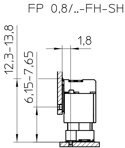
FP 0,8/..-MV-SH 2,65
