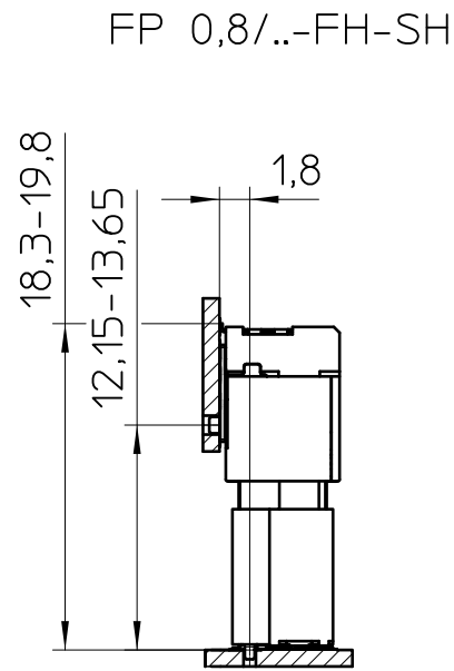
FP 0,8/..-MV-SH 8,65
