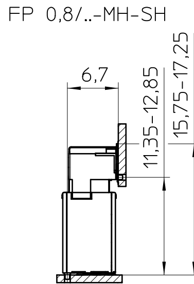
FP 0,8/..-FV-SH 10,85
