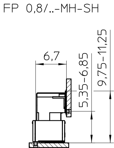
FP 0,8/..-FV-SH 4,85
