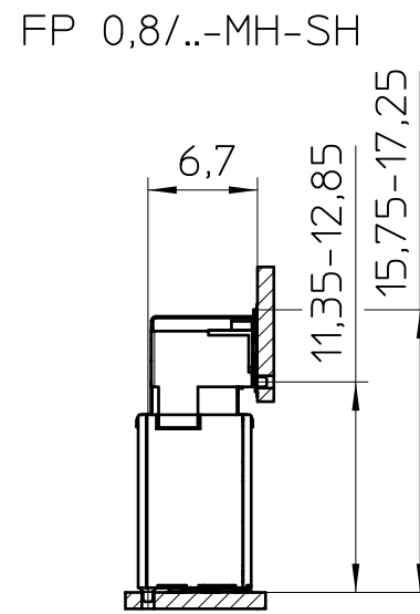
FP 0,8/..-FV-SH 10,85
