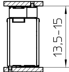
FP 0,8/..-FV-SH 10,85
